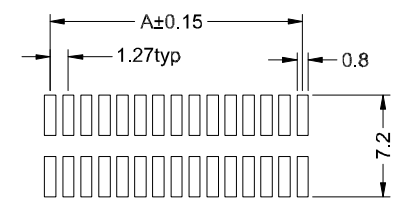
P.C.Board Layout
