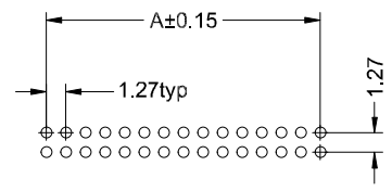
P.C.Board Layout
